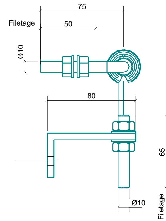
Coupe A - A 1:2
